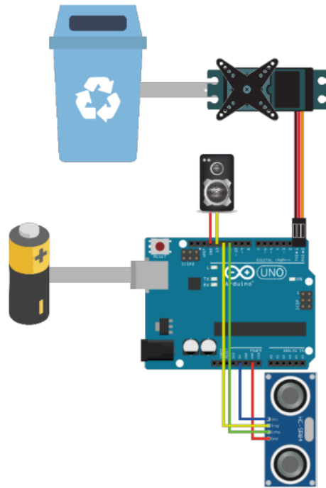
Gambar 4 Perancangan Rangkaian Smart Trash bin
