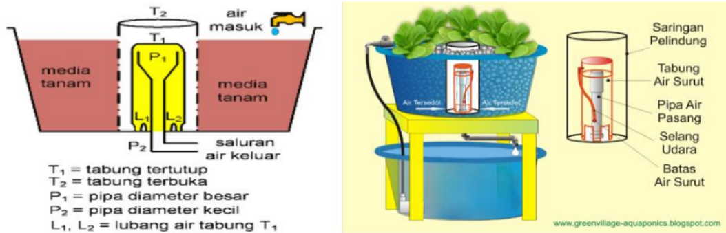
Gambar 2. Prinsip Kerja Bell-Siphon
