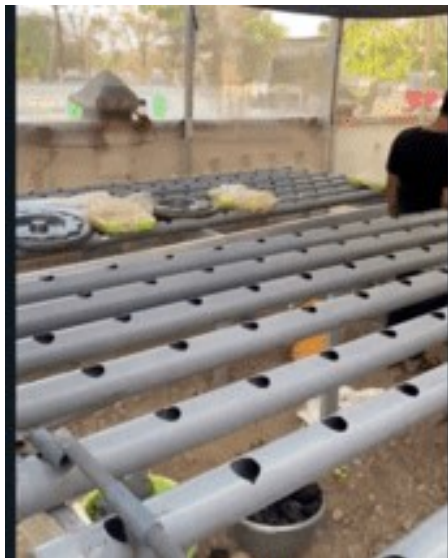
Gambar 5. Desain Prototipe instalasi Sistem hidroponik
