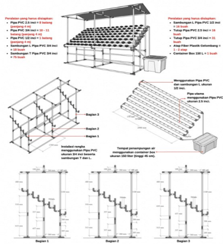
Gambar 5. Desain Prototipe instalasi Sistem hidroponik
